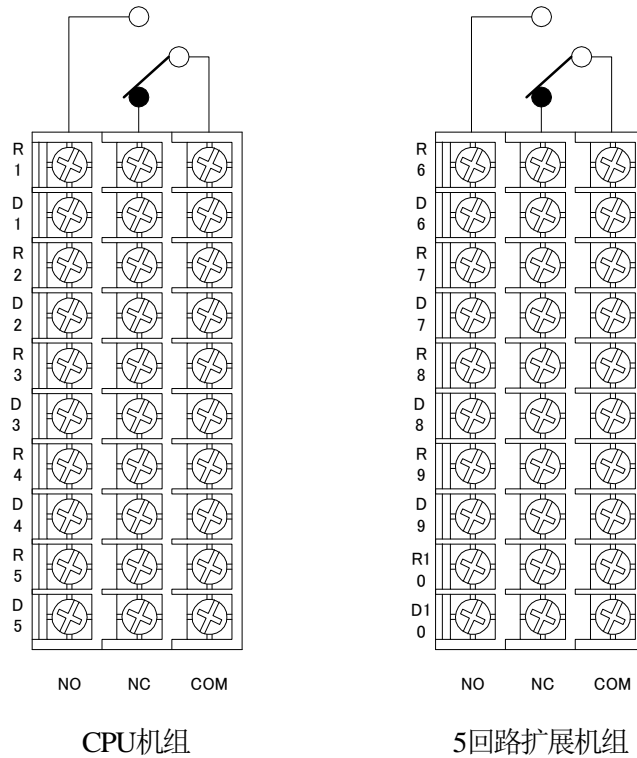
图-5.个别控制输出接点
