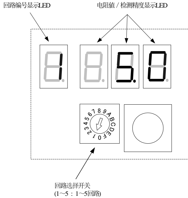
图-9.电阻值 / 检测精度显示部
