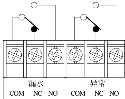
图-4.总括控制输出接点
