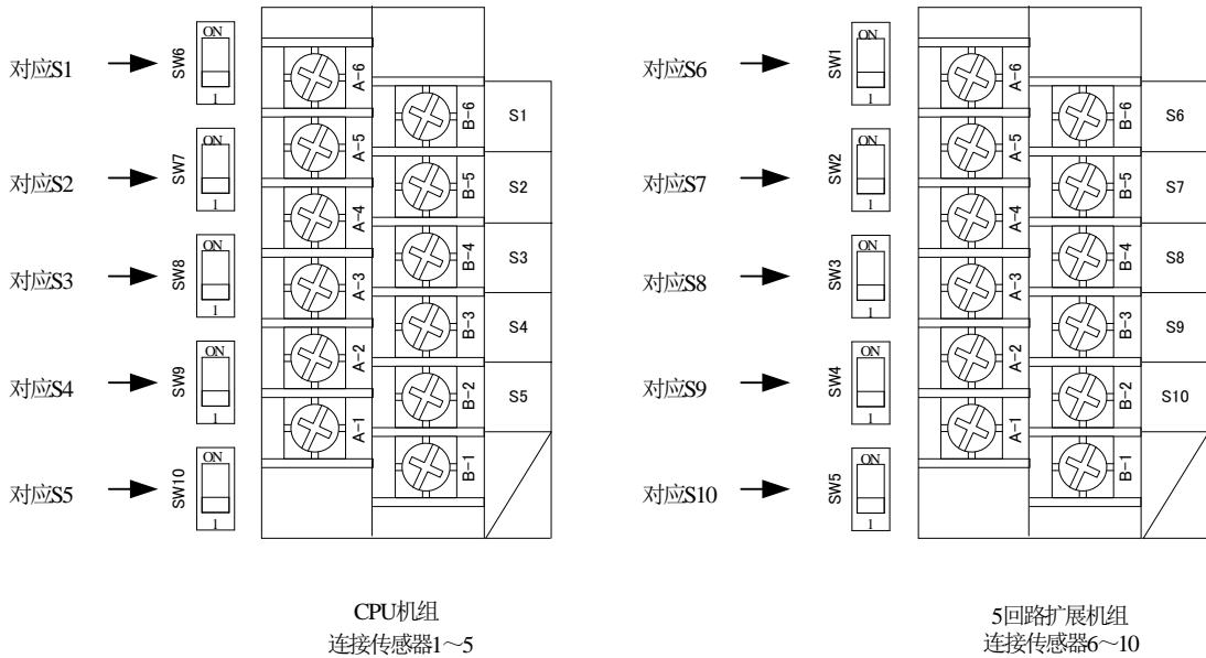
图-3.传感器端子座
