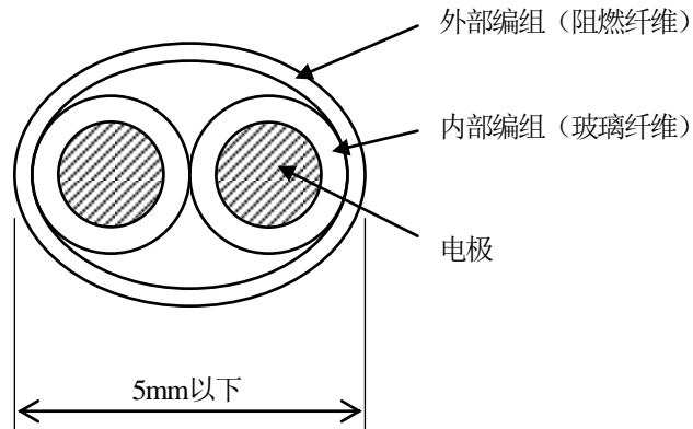
图-2.FR-AD传感器断面图
